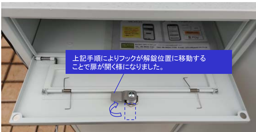
扉が開きました。 (開く際は扉はマグネットで固定されていますので強めに手前に引いてください)
