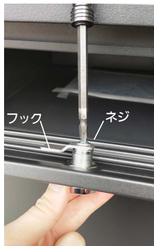
ネジを外し、フックを外す
