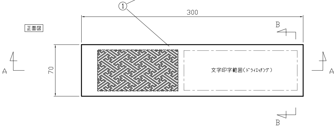
背面図
