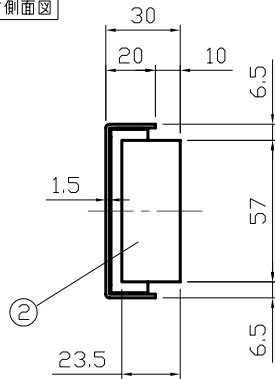
右側面図
