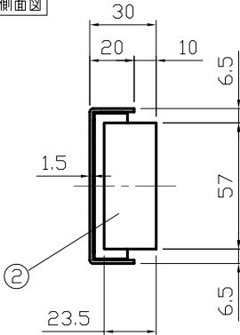
右側面図
