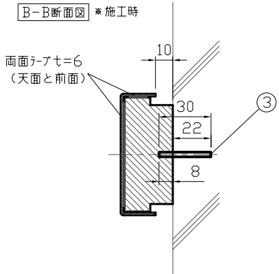
B-B断面図 ※施工時
