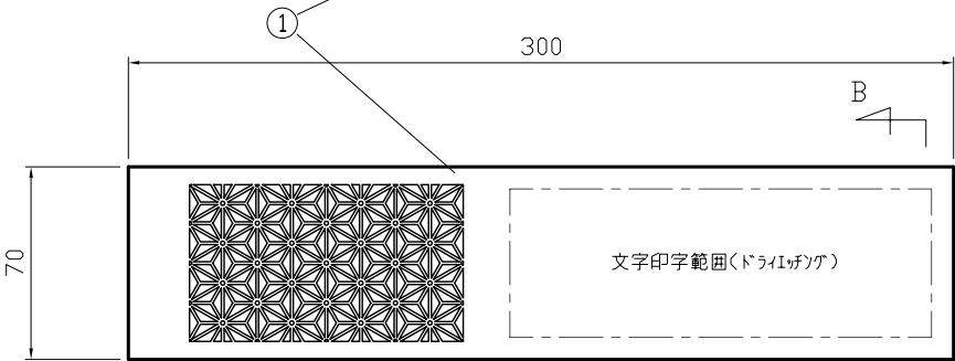
正面図
