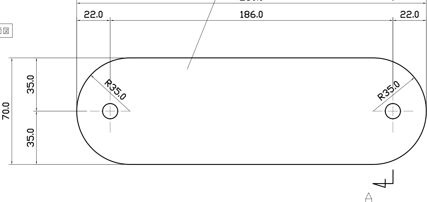
背面図
