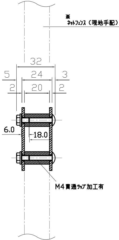
A-A断面図
