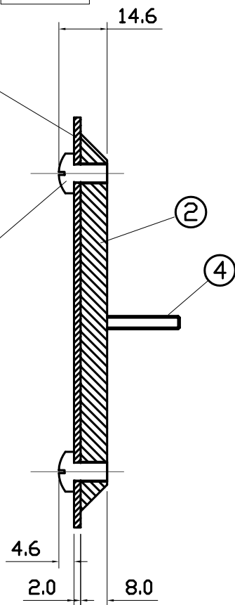
A-A断面図
