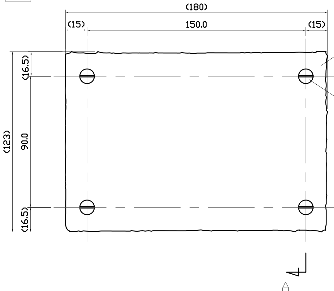
正面図
