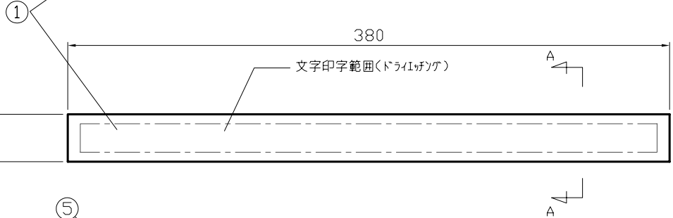
正面図
