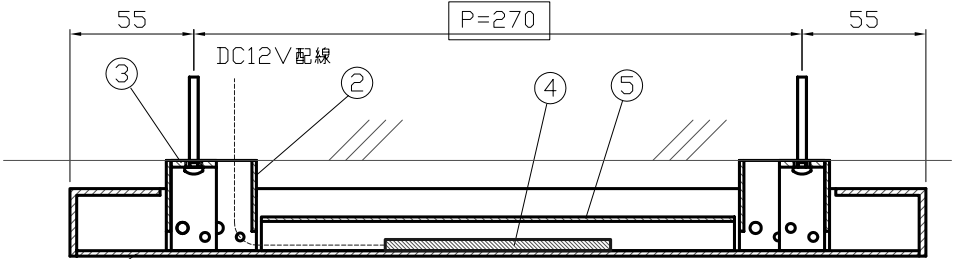
B-B断面図 ※施工時
