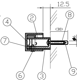
A-A断面図 ※施工時
