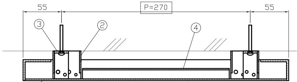
B-B断面図 ※施工時
