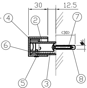
A-A断面図 ※施工時
