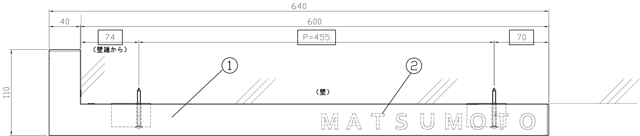
右側面図
